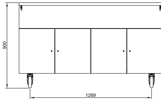
Edestä
